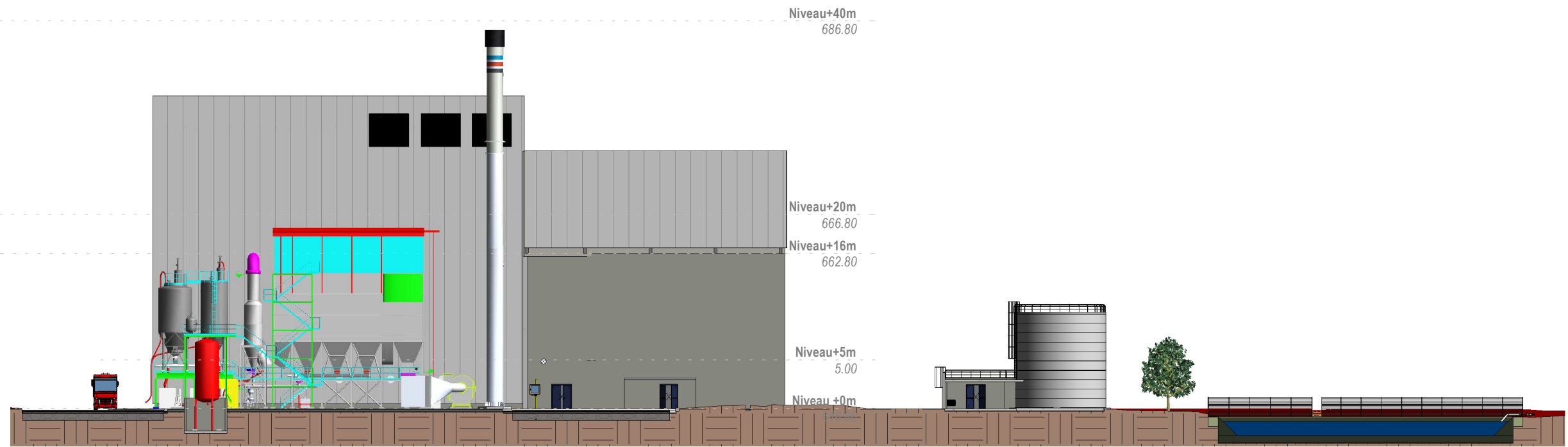
1 Coupe 1-1 Ech : 1 : 500
