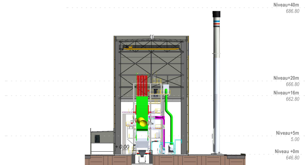
2 Coupe 2-2 Ech : 1 : 500
